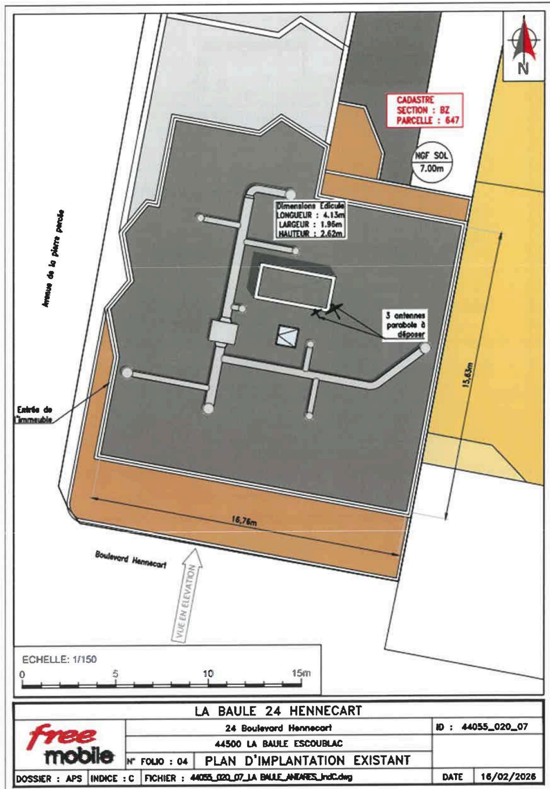
PLAN DE MASSE EXISTANT
